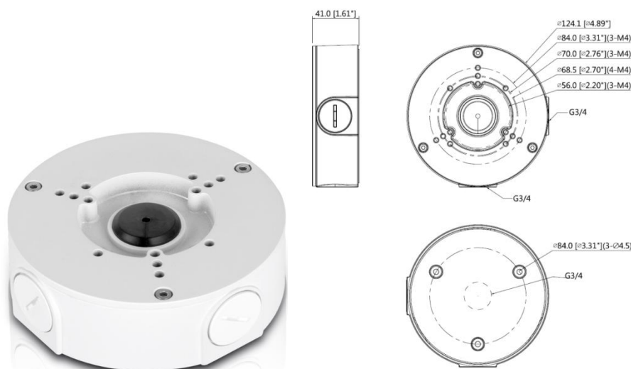
Рисунок 5.3 — Монтажная коробка BR-204
