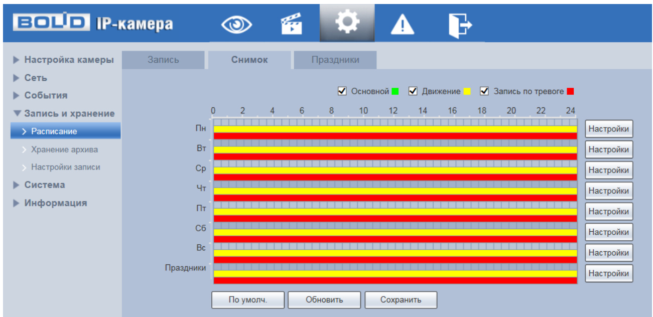
Рисунок 7.88 — Вкладка «Снимок»
