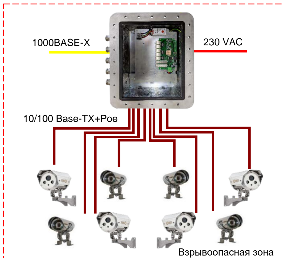
Рисунок 1. Типовая схема подключения коммутатора по оптическому кабелю
