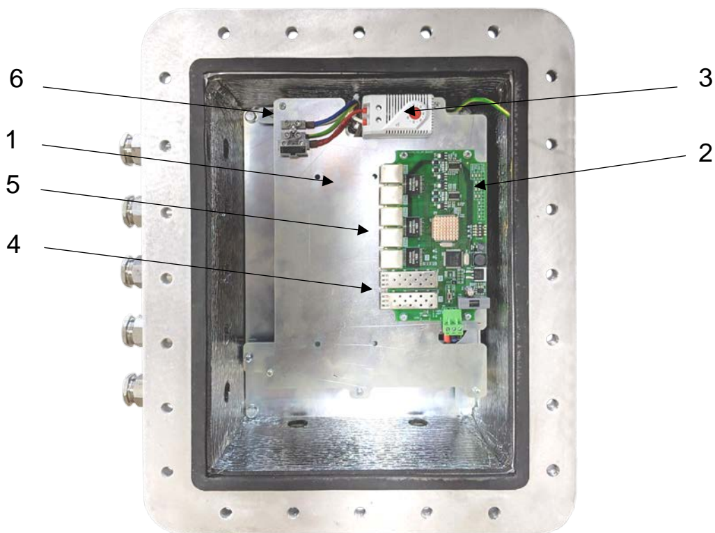
Рисунок 6. Расположение составных частей Релион-SW-EXD-A-2G-8PoE+ 1 – Источник питания; 2 – Индикаторы состояния портов коммутатора; 3 – термостат; 4 – SFP 100/1000BASE-X порт коммутатора; 5 – 10/100 Base-TX порты коммутатора с поддержкой PoE; 6 – предохранитель.
