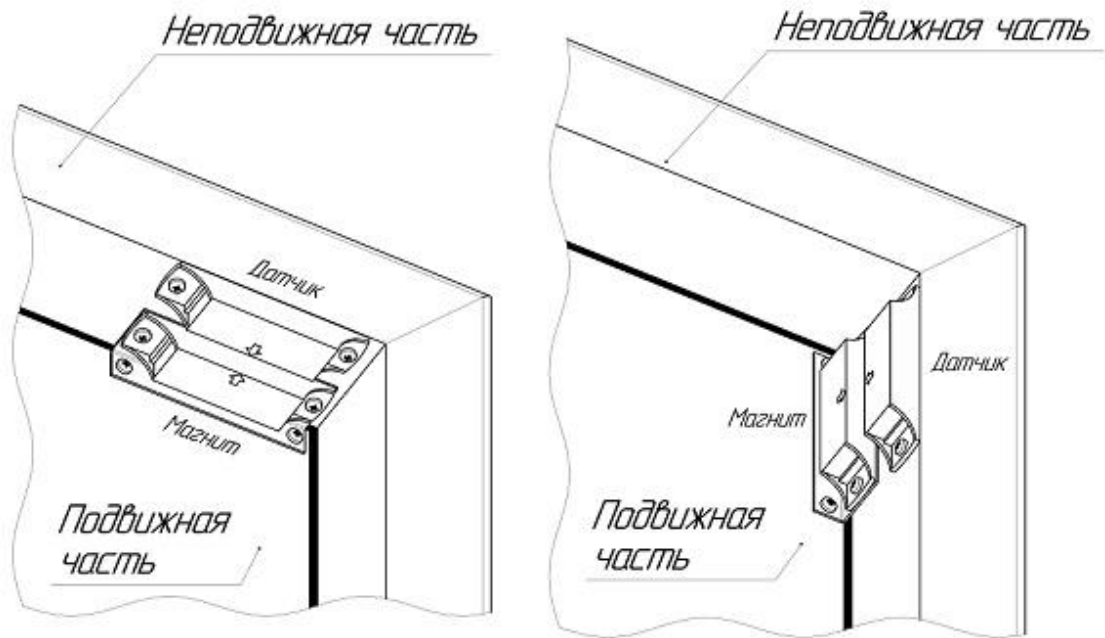
Рис.2. Вариант крепления кронштейна К-26 к подвижной поверхности охраняемой конструкции
