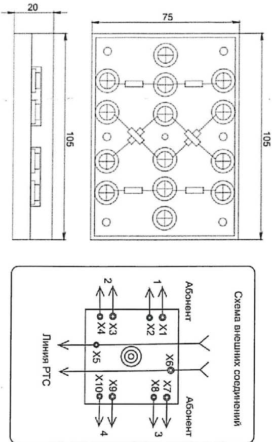
Рис.1 КОРОБКА КРА-4
